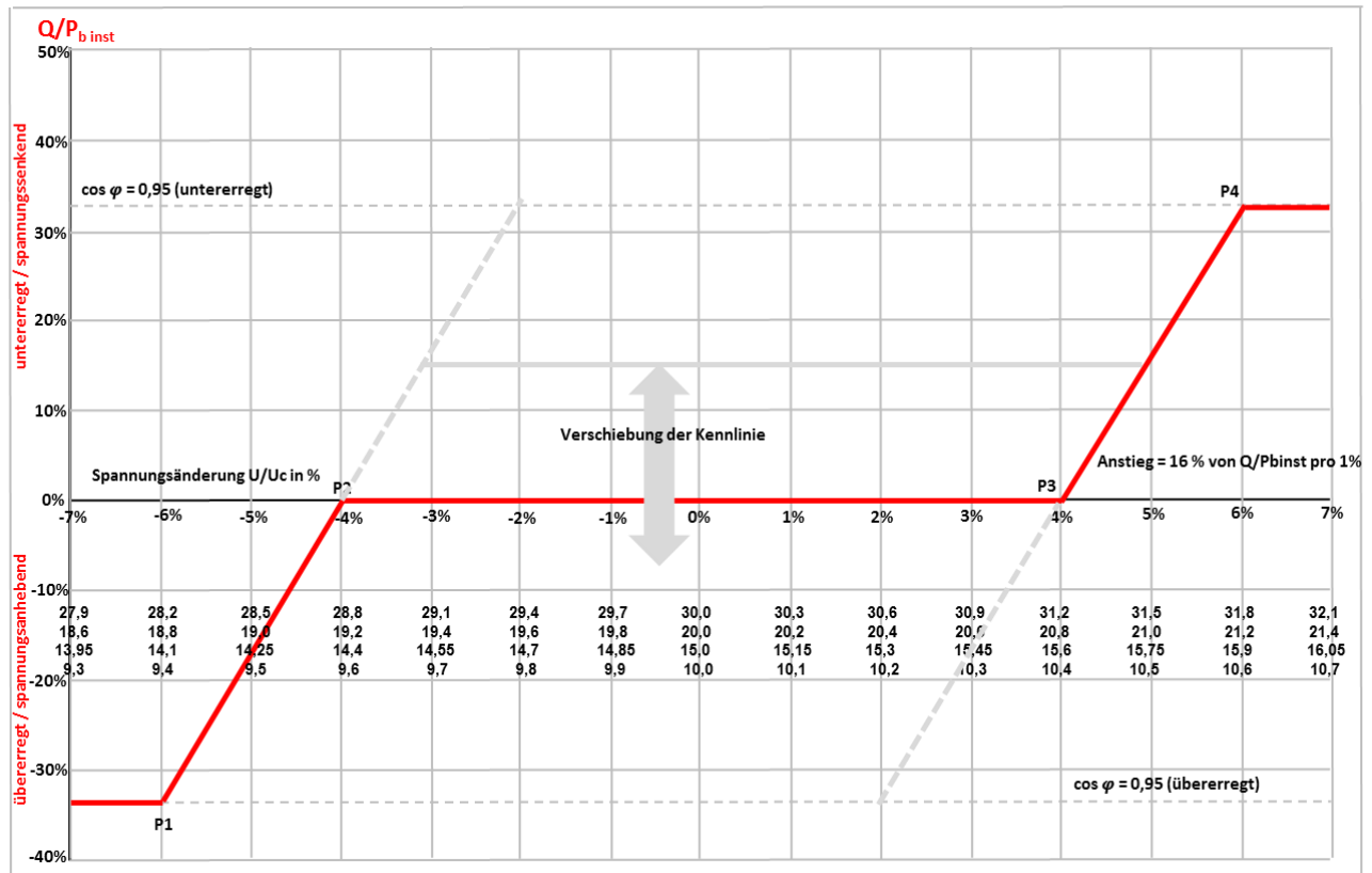
Abb. 17: Standard-Kennlinie Blindleistung mit Spannungsbegrenzungsfunktion, ehemals Bild 10.4
