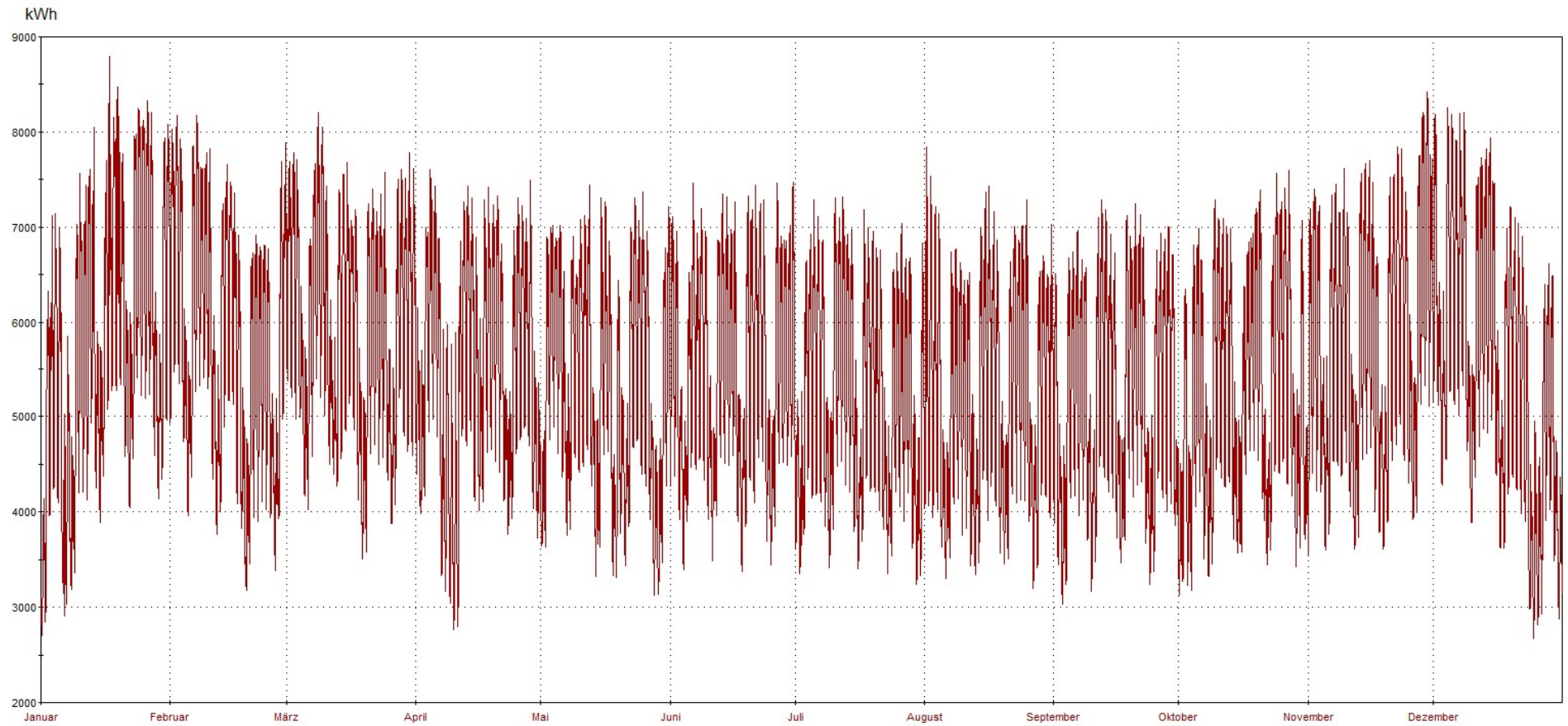
Jahreshöchstlast 35.189 kW, 17.01.2023 09:15 Uhr - Lastverlauf als viertelstündliche Leistungsmessung
