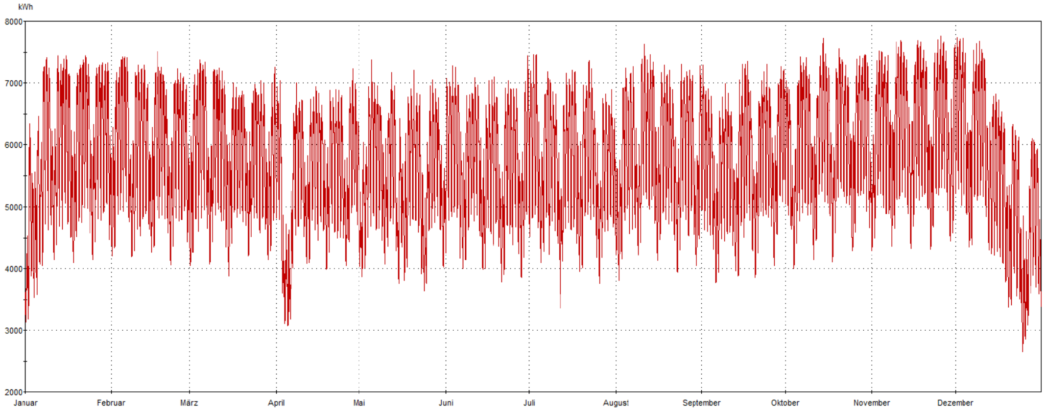
Jahreshöchstlast 31.048 kW, 25.11.2015 17:15 Uhr - Lastverlauf als viertelstündliche Leistungsmessung
