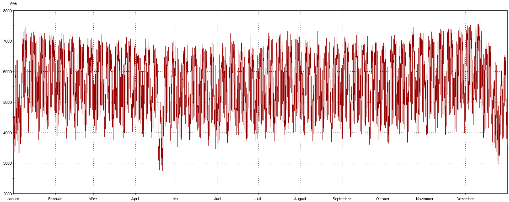
Jahreshöchstlast 30.746 kW, 03.12.2014 17:15 Uhr - Lastverlauf als viertelstündliche Leistungsmessung
