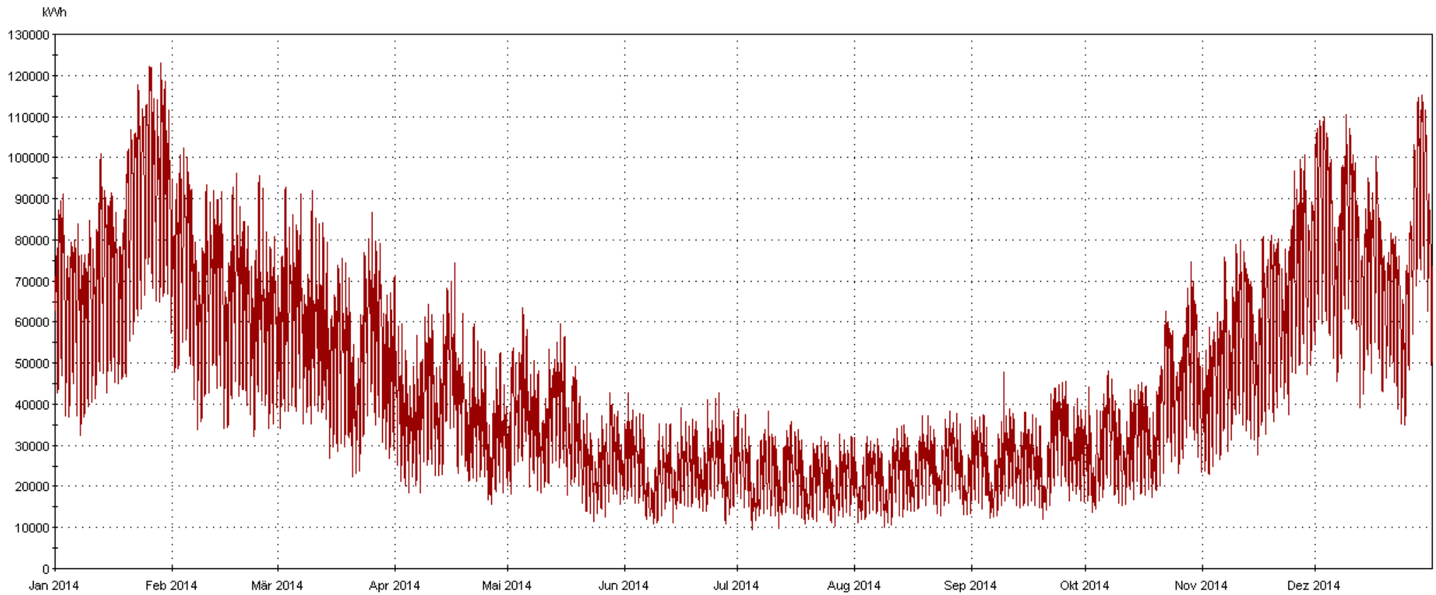
Jahreshöchstlast 123.030 kW - Lastverlauf als stündliche Leistungsmessung (Maximum am 29.01.2014 09:00 Uhr)
