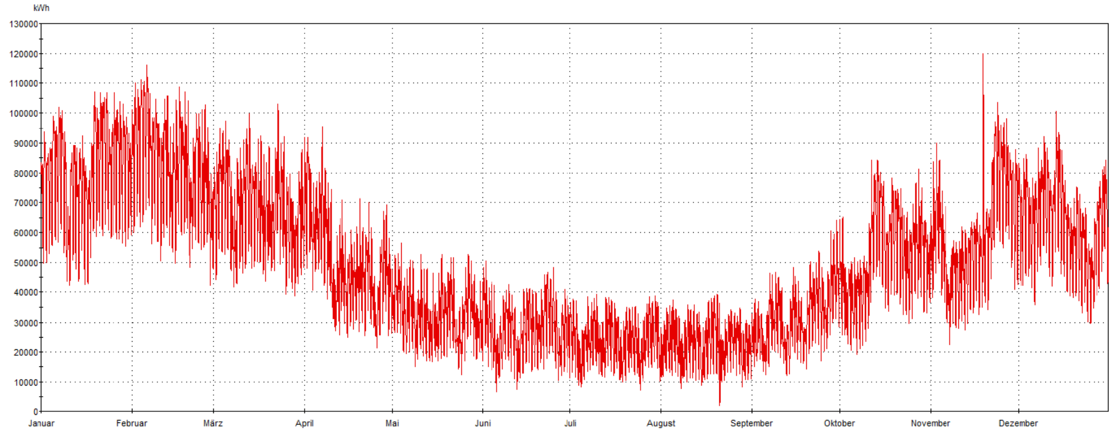
Jahreshöchstlast 120.661 kW - Lastverlauf als stündliche Leistungsmessung (Maximum am 19.11.2015 09:00 Uhr)
