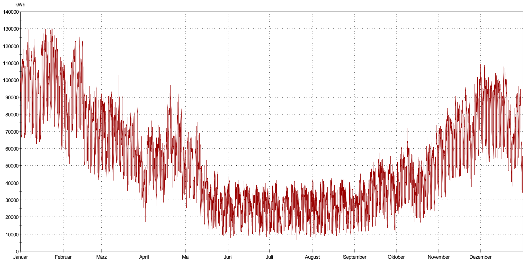
Jahreshöchstlast 130.445 kW - Lastverlauf als stündliche Leistungsmessung (Maximum am 23.01.2017 17:00 Uhr)
