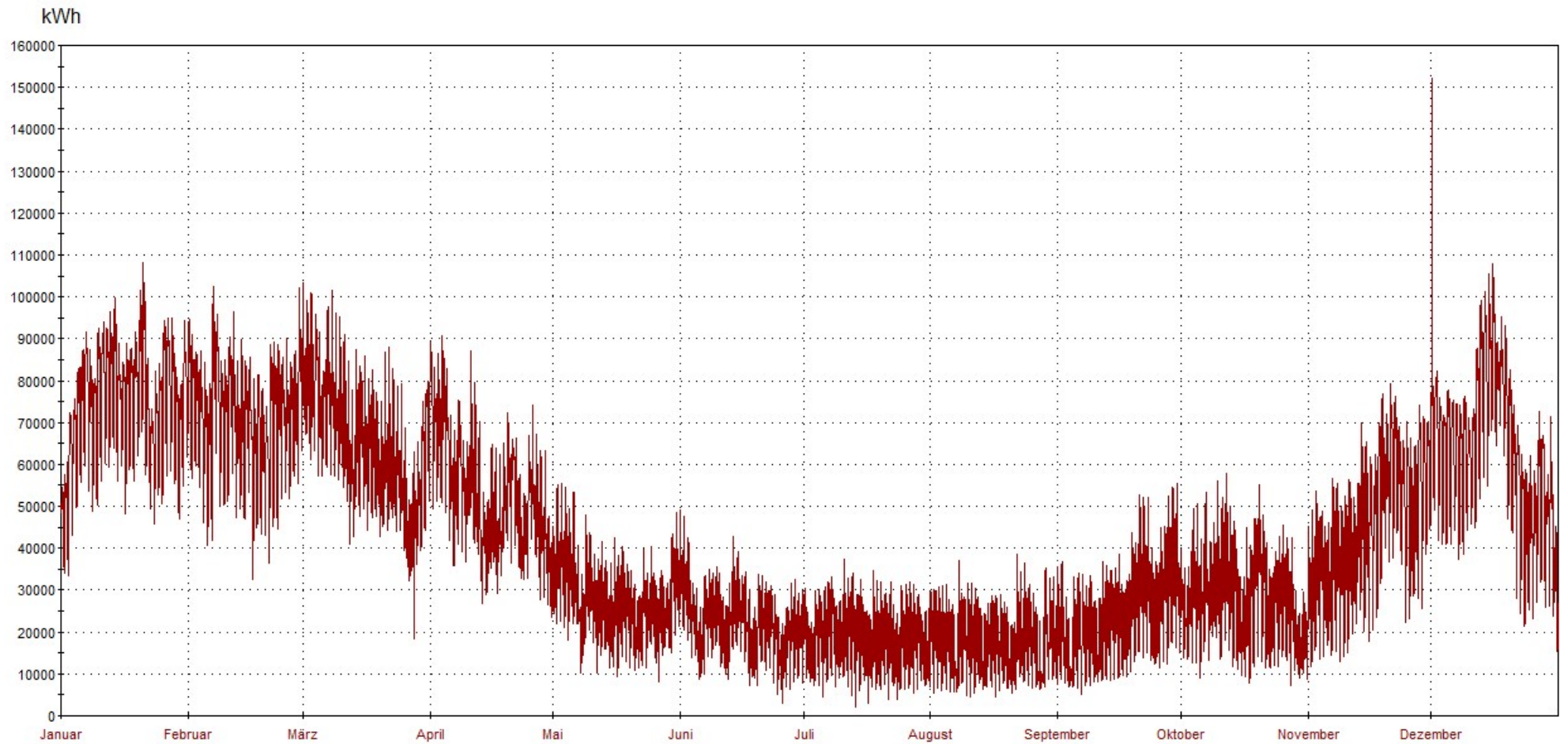
Jahreshöchstlast 152.285 kW - Lastverlauf als stündliche Leistungsmessung ( Maximum am 01.12.2022 10:00 Uhr )
