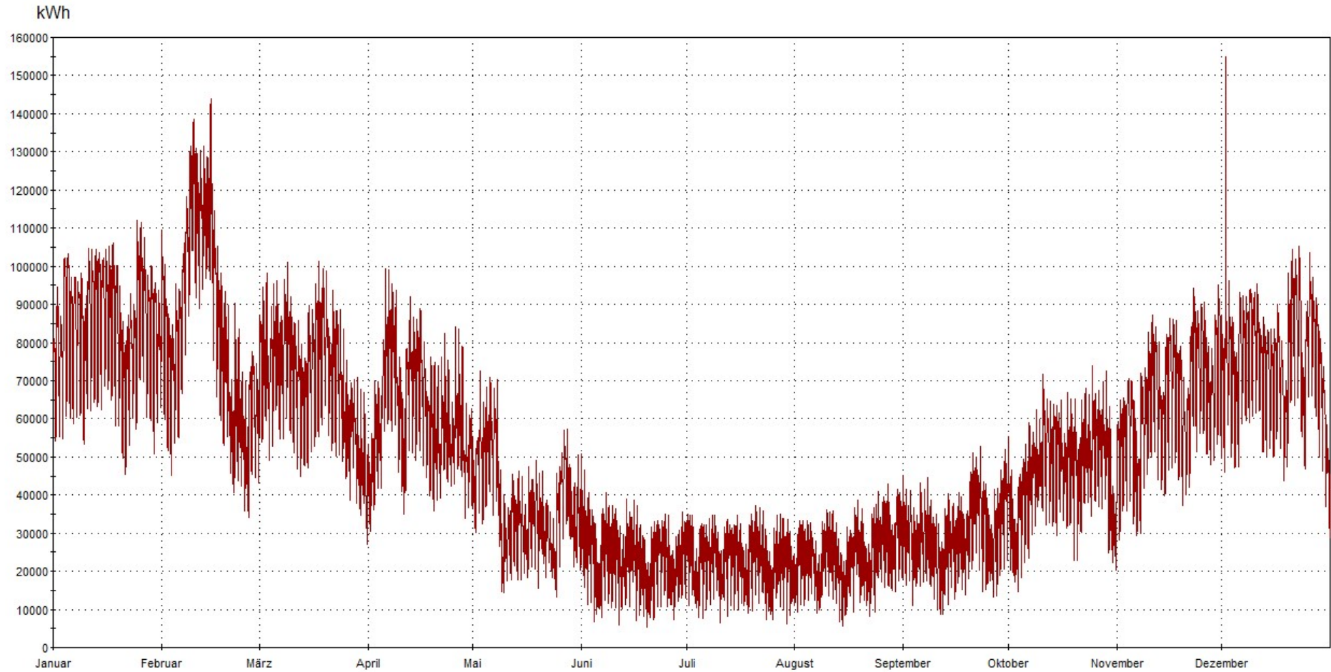
Jahreshöchstlast 155.021 kW - Lastverlauf als stündliche Leistungsmessung ( Maximum am 02.12.2021 10:00 Uhr )
