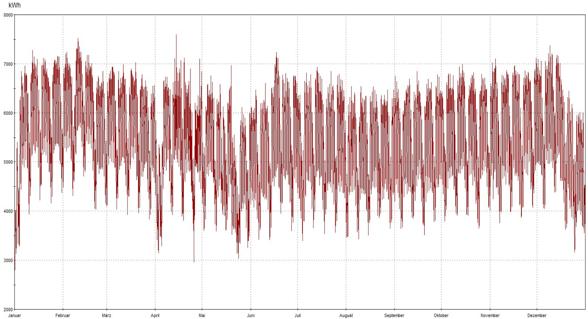
Jahreshöchstlast 30.381 kW, 14.04.2021 10:00 Uhr - Lastverlauf als viertelstündliche Leistungsmessung
