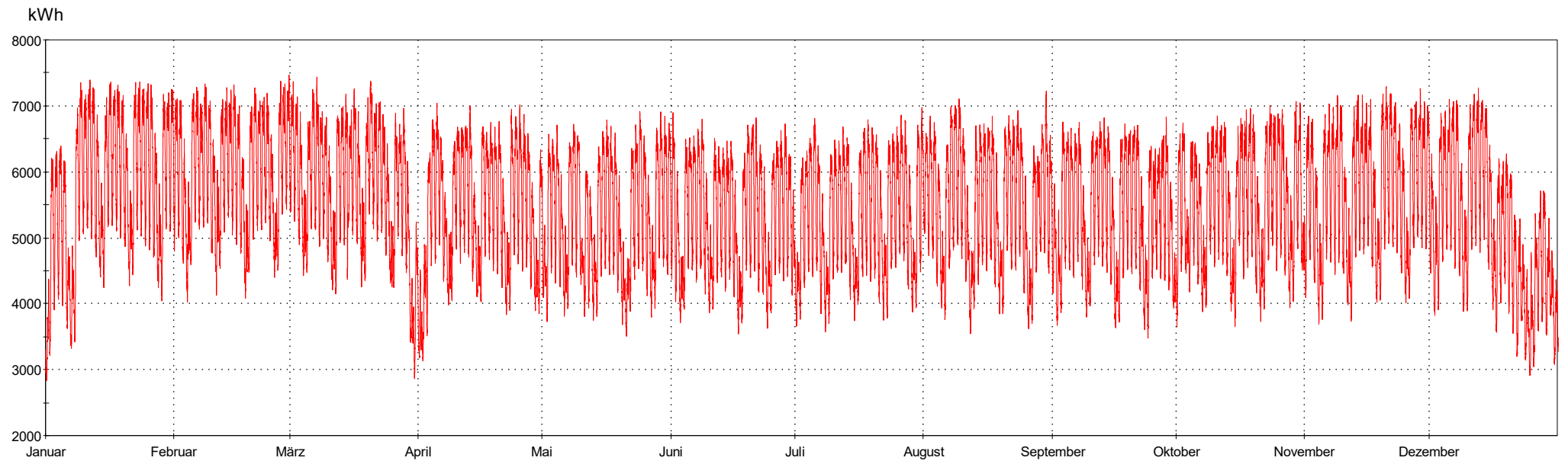
Jahreshöchstlast 29.857 kWh, 28.02.2018 18:15 Uhr - Lastverlauf als viertelstündliche Leistungsmessung
