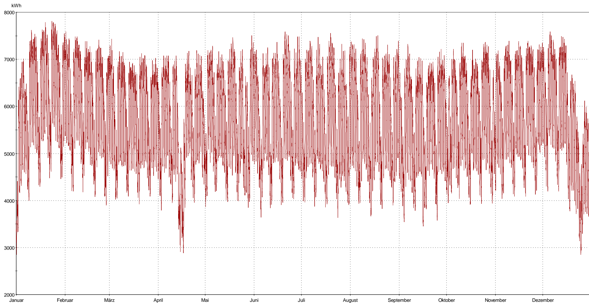
Jahreshöchstlast 31.245 kW, 23.01.2017 17:15 Uhr - Lastverlauf als viertelstündliche Leistungsmessung
