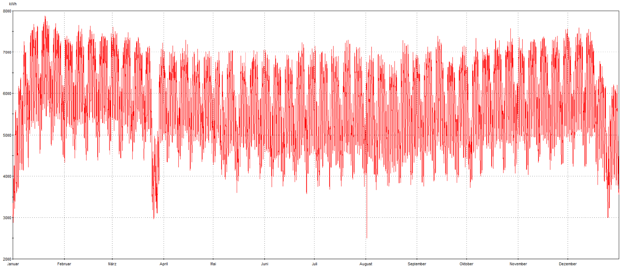
Jahreshöchstlast 31.522 kW, 20.01.2016 11:15 Uhr - Lastverlauf als viertelstündliche Leistungsmessung
