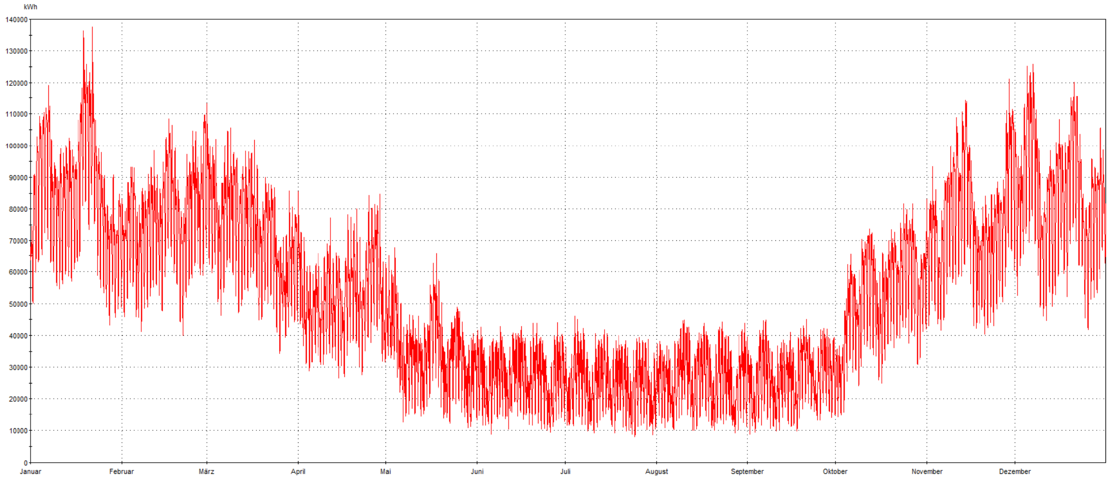
Jahreshöchstlast 137.582 kW - Lastverlauf als stündliche Leistungsmessung (Maximum am 22.01.2016 08:00 Uhr)
